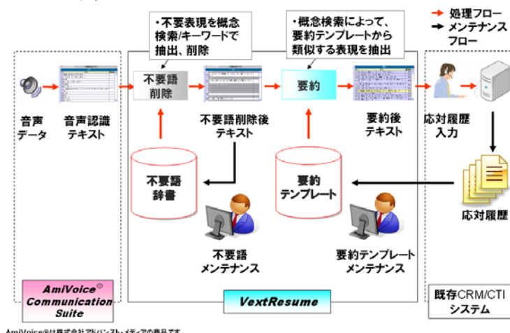
図1: VextResume の処理フロー
